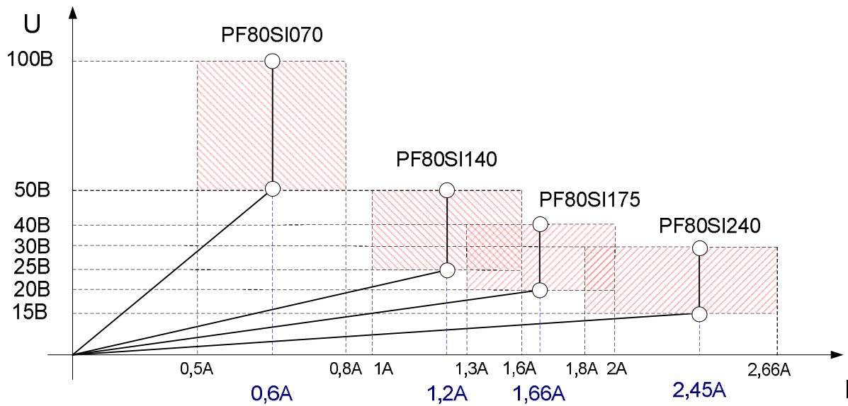
Рис. 1 Вольт-амперная характеристика. Заштрихованной областью показаны рабочие зоны токов и напряжений.
