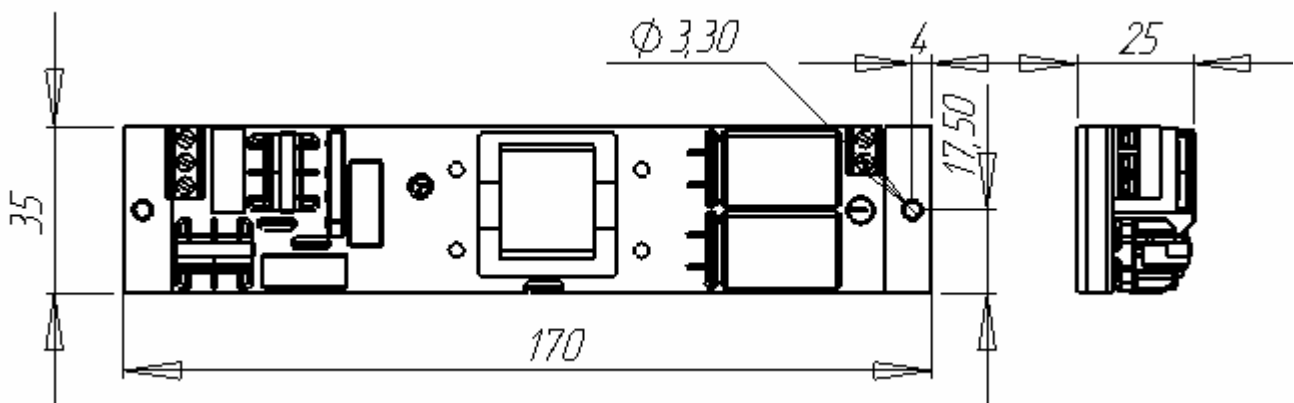
Рис. 3 Размеры блока в исполнении с заливкой
