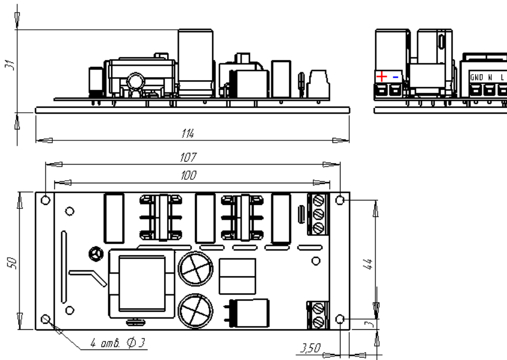
Рис. 3 Размеры блока в исполнении на алюминиевой плите с клеммниками
