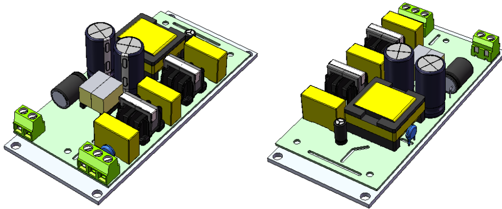
Рис. 2 Блок в исполнении на алюминиевой плите с клеммниками
